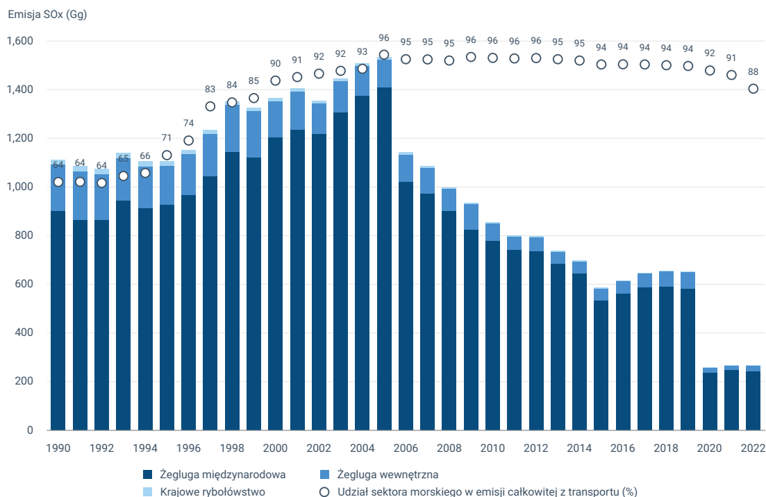
Rysunek 5 Emisja SOx z sektora morskigo (Gg) i jej udział w emisji całkowitej z transportu (%) w latach 1990–2022 w UE-27
