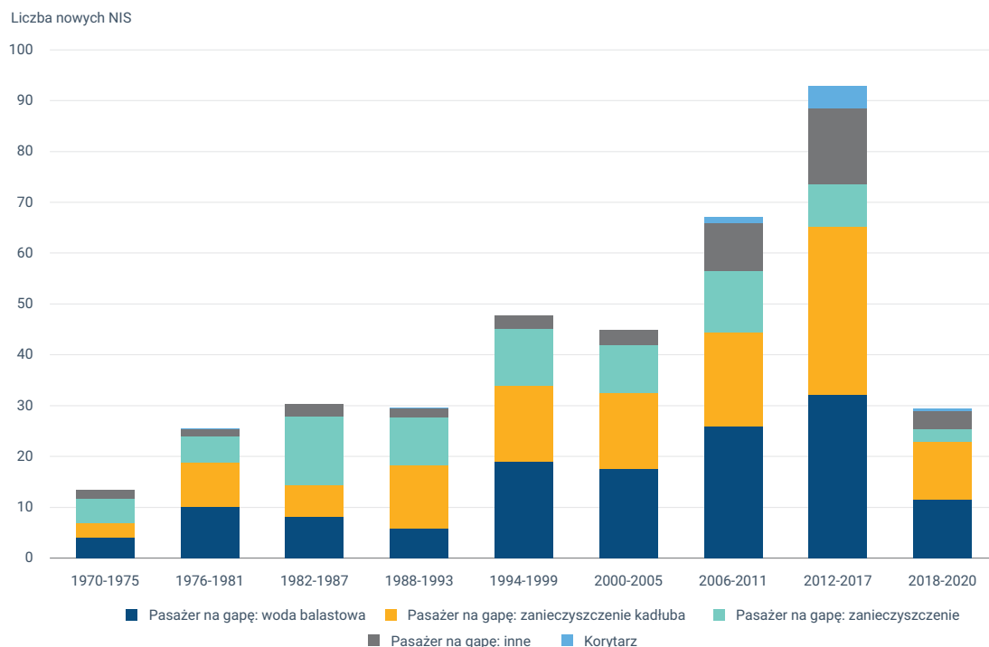
Rysunek 11 Liczba nowych gatunków nierodzących (NIS) w europejskich morzach regionalnych wprowadzonych przez transport morski, w cyklach sześcioletnich
