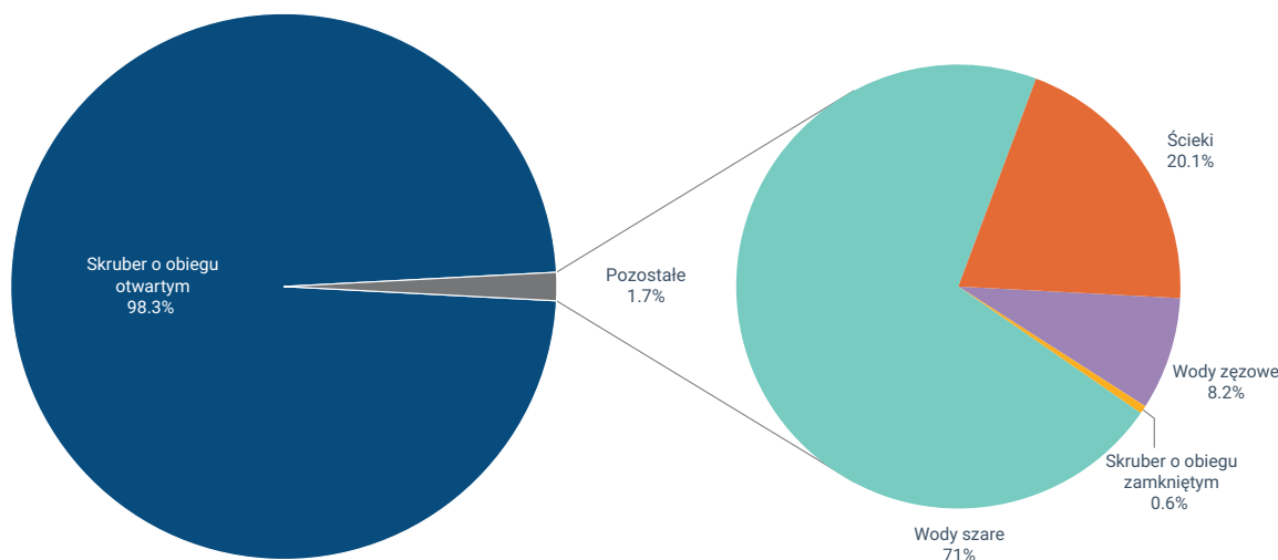
Rysunek 8 Skład zrzutów do wód europejskich w 2023 r. (po lewej) oraz przybliżenie składu zrzutów z wyłączeniem zrzutów ze skruberów o obiegu otwartym (po prawej)
