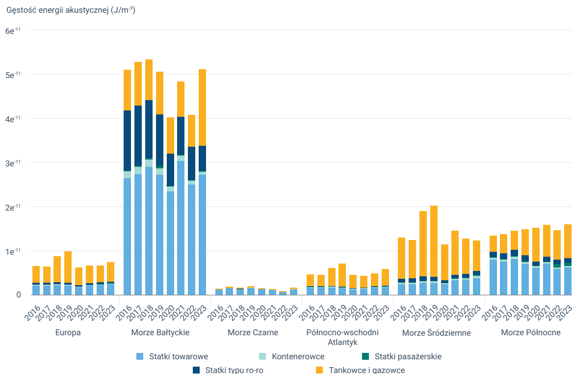
Rysunek 9 Gęstość energii akustycznej URN przy 63 Hz (Europa, lewy skraj wykresu, i morza regionalne) w latach 2016–2023
